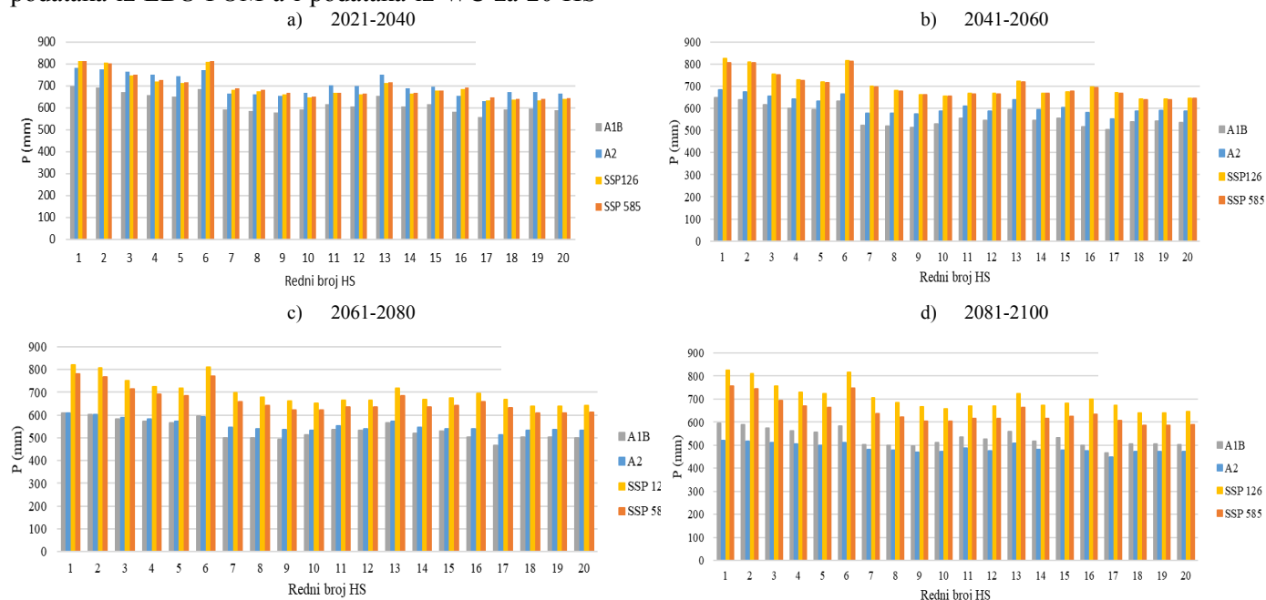
Slika 18 – Vrednosti padavina na slivovima HS dobijenih na osnovu podataka iz EBU-POM-a i WC za četiri perioda predikcije
