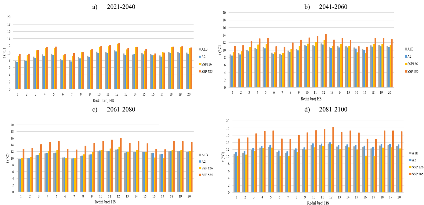
Slika 19– Vrednosti temperaura na slivovima HS dobijenih na osnovu podataka iz EBU-POM-a i WC za četiri perioda predikcije
